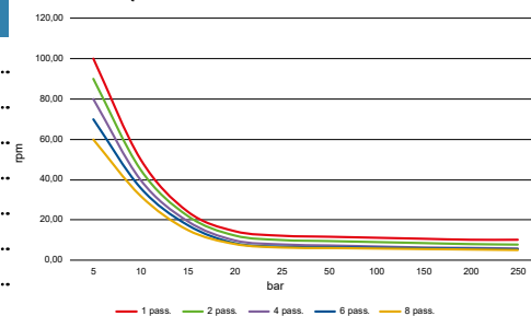
Prędkość obrotowa w zależności od ilości kanałów
